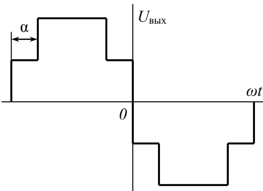
Рис. 4. Кривая выходного напряжения трехуровневого преобразователя.
