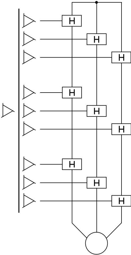
Рис. 10. Упрощенная схема каскадного преобразователя на H-ячейках.
