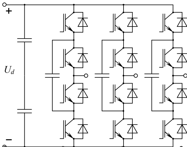
Рис. 7. Трехуровневый преобразователь с плавающими конденсаторами.
