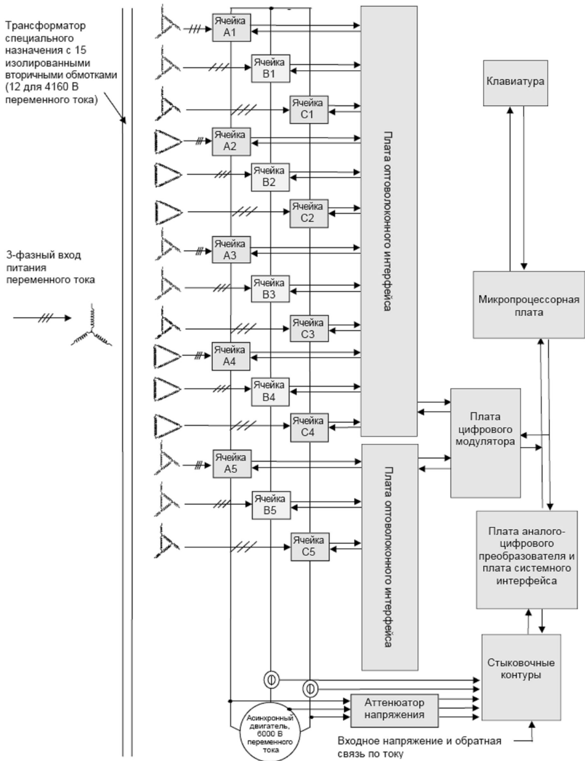
Рис. 12. Структурная схема системы частотного регулирования электродвигателей на основе каскадного преобразователя частоты на H-мостовых ячейках.
