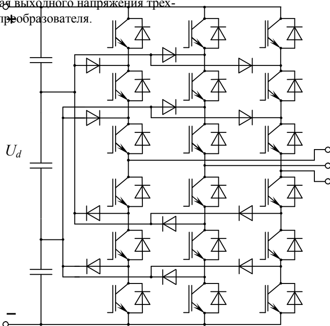
Рис. 5. 4-уровневый преобразователь с привязкой средней точки.
