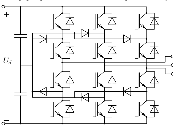
Рис. 2. Трехуровневый преобразователь с привязкой средней точки.
