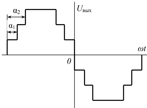
Рис. 6. Кривая выходного напряжения четырехуровневого преобразователя.
