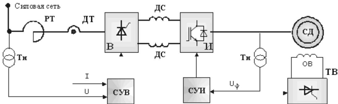
Рис. 1. Электропривод прямого преобразования ПЧСВ: В – управляемый выпрямитель; РТ – входной реактор; ДТ – датчик тока; ДС – сглаживающие дроссели; И – инвертор; СУВ – система управления выпрямителем; СУИ – система управления инвертором; Тн – измерительные трансформаторы напряжения; ТВ – тиристорный возбудитель; ОВ – обмотка возбуждения синхронного двигателя.
