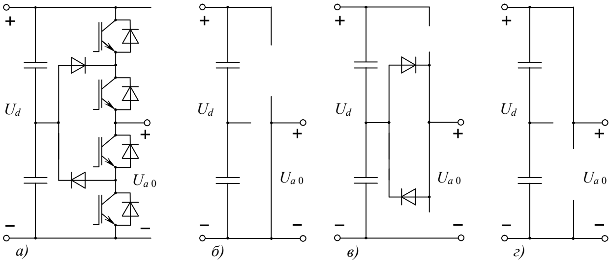
Рис. 3. Диаграммы состояния фазы трехуровневого преобразователя с привязкой средней точки: а) схема одной фазы; б) состояние U_{a0} = 0 ; в) состояние U_{a0} = 0,5U_d ; з) состояние U_{a0} = U_d .
