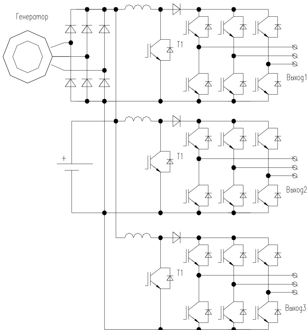
Рис. 1. Преобразователь статический М-ПТЕ-22-У1
