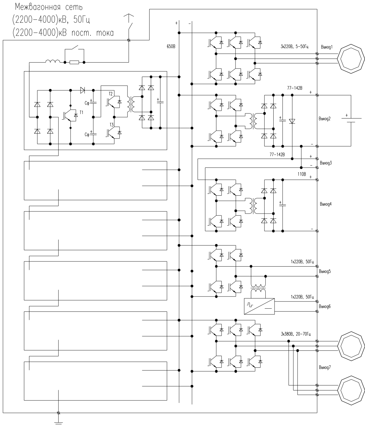
Рис. 3. Преобразователь статический БЭВ
