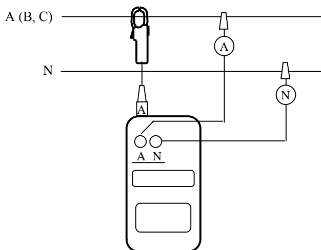
Рис. 2. Схема подключения прибора для измерения тока, напряжения, частоты, активной, реактивной, полной мощности и коэффициента мощности в однофазной сети
