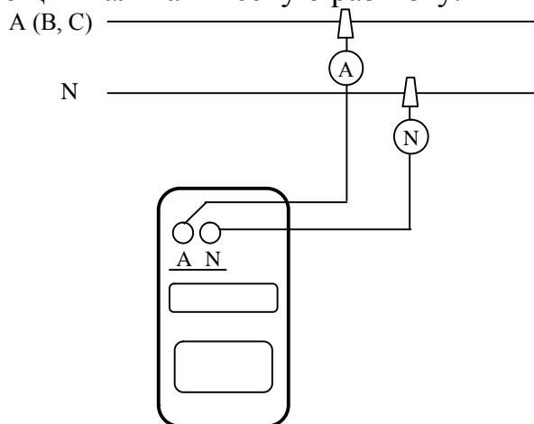
Рис. 4. Схема подключения прибора для измерения фазового напряжения и частоты сети
